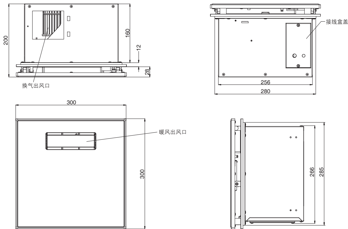
产品尺寸图 (单位：毫米)
