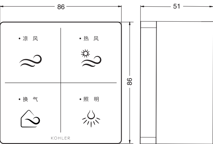
墙装开关尺寸图
